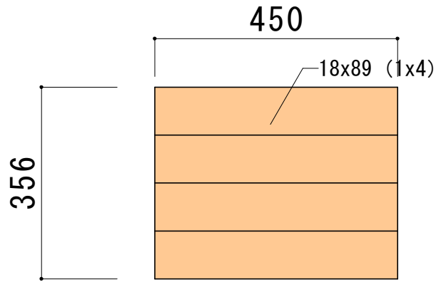
平面図 1/10
