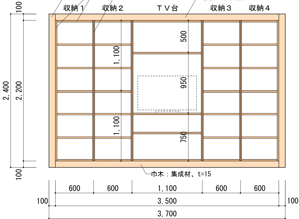
立面図 1/30
