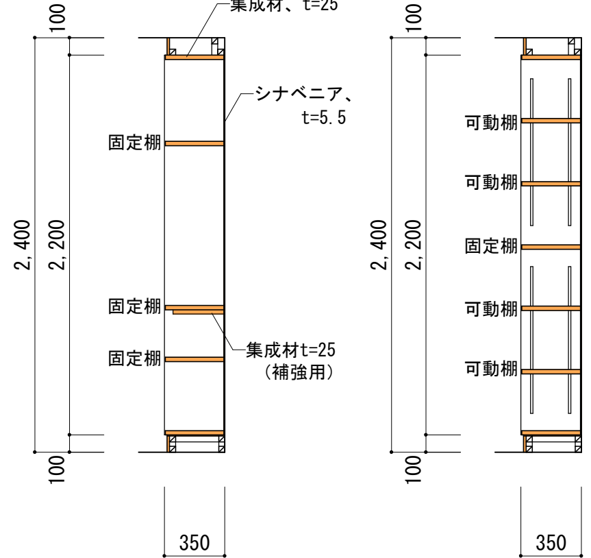
断面図 1/30
